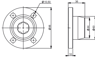
6 FREZE 4 DELİKLİ FLANŞ Ø98 6 SPLINA 4 HOLES
